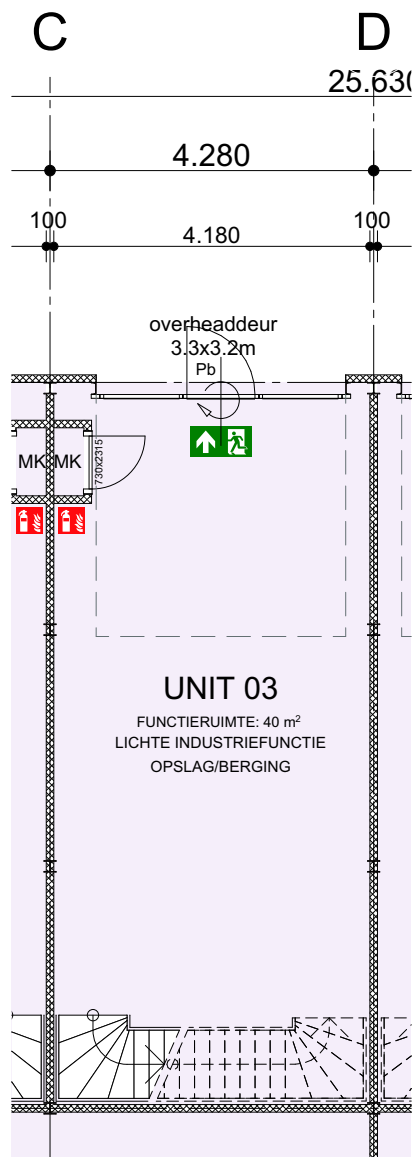
BEGANEGROND (0.00)
